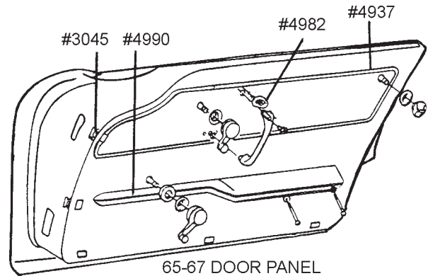
65-67 DOOR PANEL
